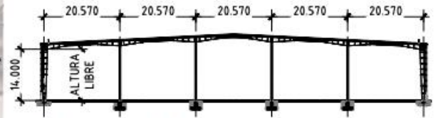
CORTE TRANSVERSAL
